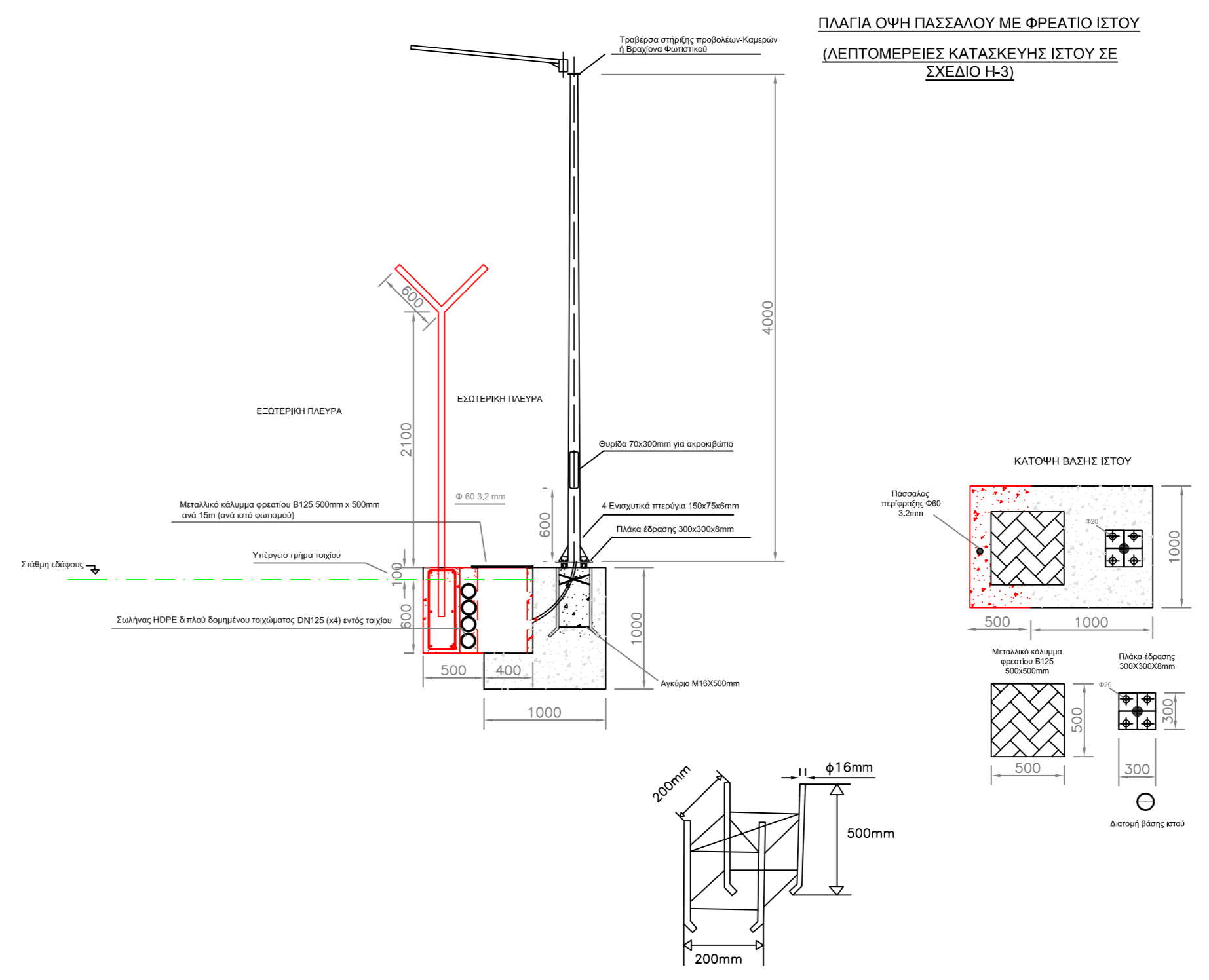
ΤΟΜΗ ΚΑΤΑΣΚΕΥΗΣ ΕΣΩΤΕΡΙΚΗΣ ΠΕΡΙΜΕΤΡΙΚΗΣ ΠΕΡΙΦΡΑΞΗΣ ΠΕΡΙΟΧΗΣ 1 ( ΕΞΩ Π1) ΚΑΤΑΣΚΕΥΗ ΣΥΝΕΧΟΥΣ ΤΟΙΧΙΟΥ ΣΚΥΡΟΔΕΜΑΤΟΣ ΚΑΙ ΙΣΤΙΟΥ ΦΩΤΙΣΜΟΥ 4m
