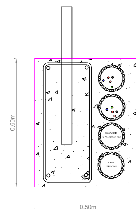
ΥΠΑΙΘΡΙΟ ΠΙΛΛΑΡ ΠΡΟΣ ΚΥΚΛΩΜΑ ΦΩΤΙΣΜΟΥ 2 και ΗΣΑ
