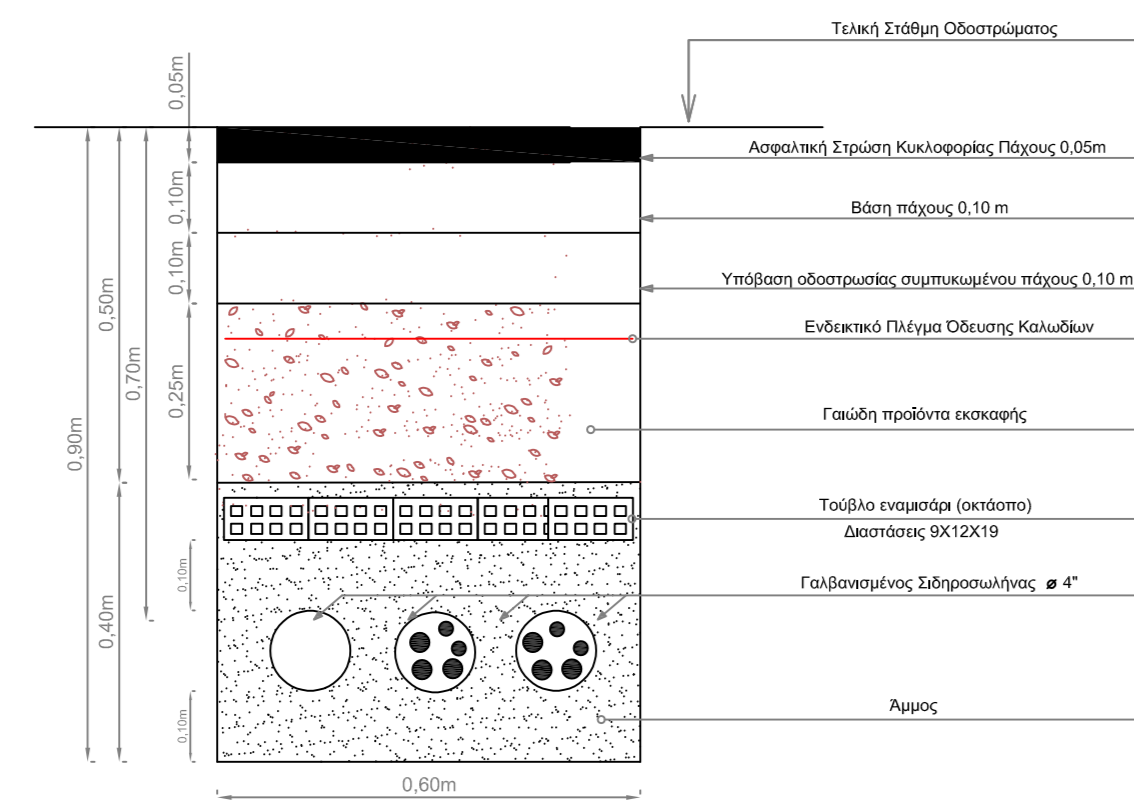
ΥΠΟΣΤΑΘΜΟΣ - ΥΠΑΙΘΡΙΟ ΠΙΛΛΑΡ (ΔΡΟΜΟΣ)
