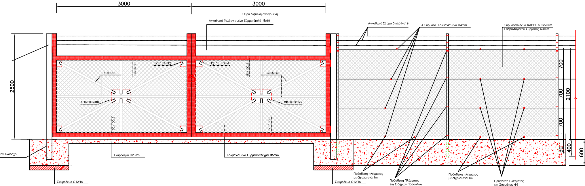
ΕΣΤΕΡΝΗ ΟΨΗ ΑΒΥΣΣΗΣ ΘΥΡΑΣ ΑΝΚΥΡΩΜΕΝΗ ΔΙΑ ΟΙΚΙΑΤΑ ΚΑΙ ΠΛΕΓΜΑΤΟΣ ΠΕΡΙΦΡΑΣΗΣ
