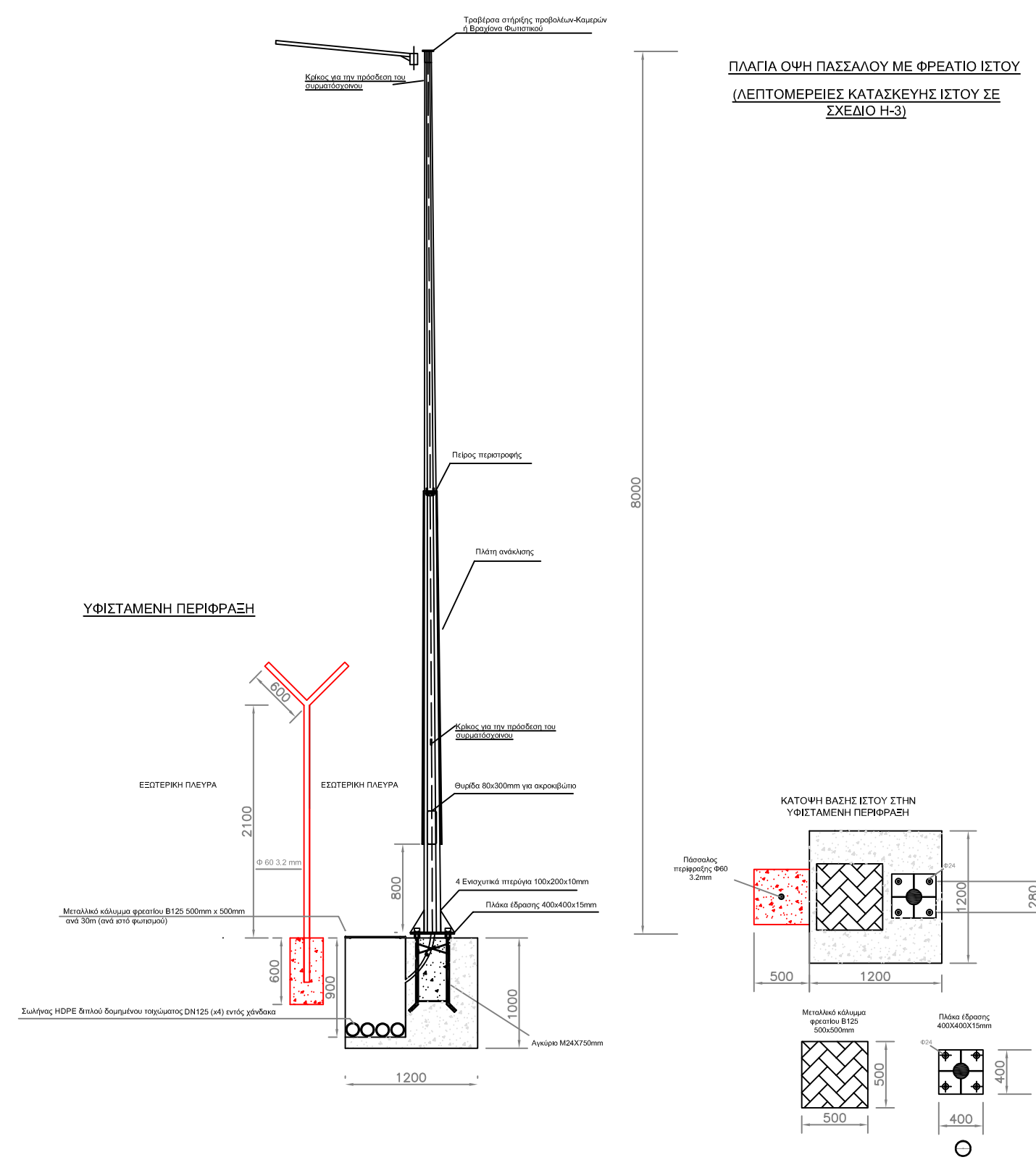
ΤΟΜΗ ΚΑΤΑΣΚΕΥΗΣ ΕΣΤΕΡΝΗΣ ΠΕΡΙΜΕΤΡΙΚΗΣ ΠΕΡΙΦΡΑΣΗΣ ΠΕΡΙΟΧΗ 1 (ΕΣΩ Π1)
