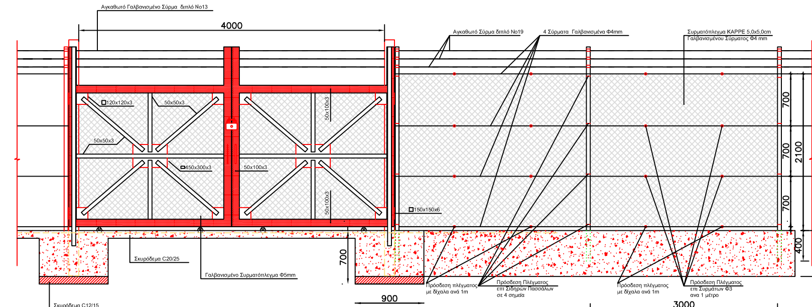
ΕΣΤΕΡΝΗ ΟΨΗ ΑΒΥΣΣΗΣ ΘΥΡΑΣ ΕΥΡΩΜΕΝΗ ΔΙΑ ΟΙΚΙΑΤΑ ΚΑΙ ΠΛΕΓΜΑΤΟΣ ΠΕΡΙΦΡΑΣΗΣ
