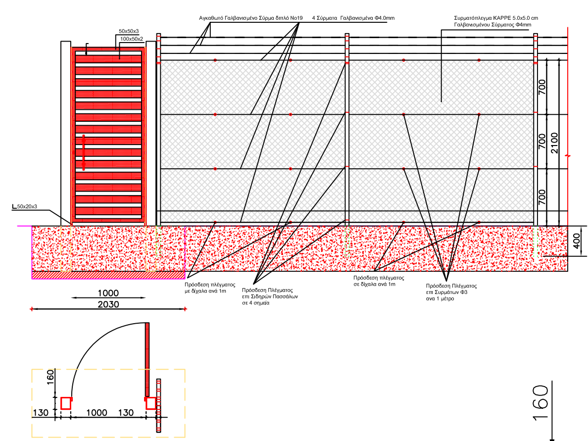
ΕΣΤΕΡΝΗ ΟΨΗ ΠΥΛΩΣ ΕΙΣΟΔΟΥ ΠΡΟΣΠΕΥΚΩ ΚΑΙ ΠΛΕΓΜΑΤΟΣ ΠΕΡΙΦΡΑΣΗΣ
