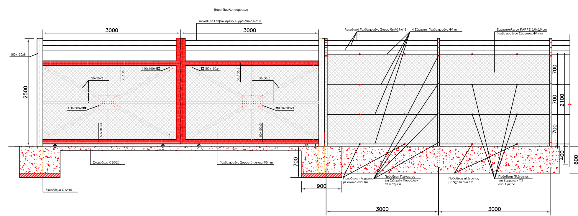
ΕΣΤΕΡΝΗ ΟΨΗ ΕΥΡΩΜΕΝΗ ΠΛΑΤΗ ΕΙΣΟΔΟΥ ΟΙΚΙΑΤΩΝ ΚΑΙ ΠΡΟΣΠΕΥΚΩ ΚΑΙ ΠΛΕΓΜΑΤΟΣ ΠΕΡΙΦΡΑΣΗΣ
