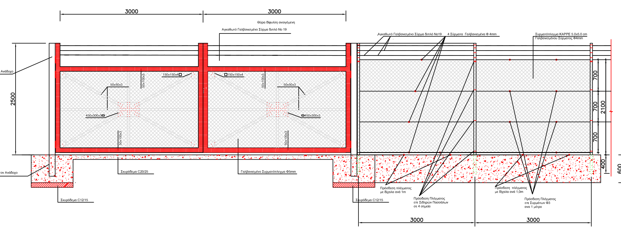
ΕΣΤΕΡΝΗ ΟΨΗ ΑΝΚΥΡΩΜΕΝΗ ΠΛΑΤΗ ΕΙΣΟΔΟΥ ΟΙΚΙΑΤΩΝ ΚΑΙ ΠΡΟΣΠΕΥΚΩ ΚΑΙ ΠΛΕΓΜΑΤΟΣ ΠΕΡΙΦΡΑΣΗΣ
