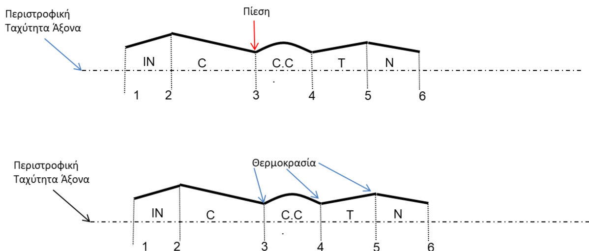
Σχήμα 1. Σχεδιάγραμμα κινητήρα με απαραίτητες θέσεις μέτρησης πίεσης και θερμοκρασίας
