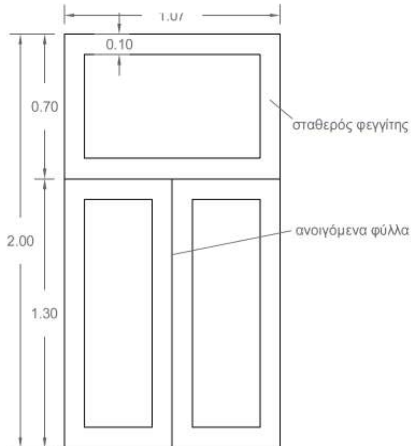
Σχέδιο 2: Διαστάσεις παραθύρου προθαλάμου
