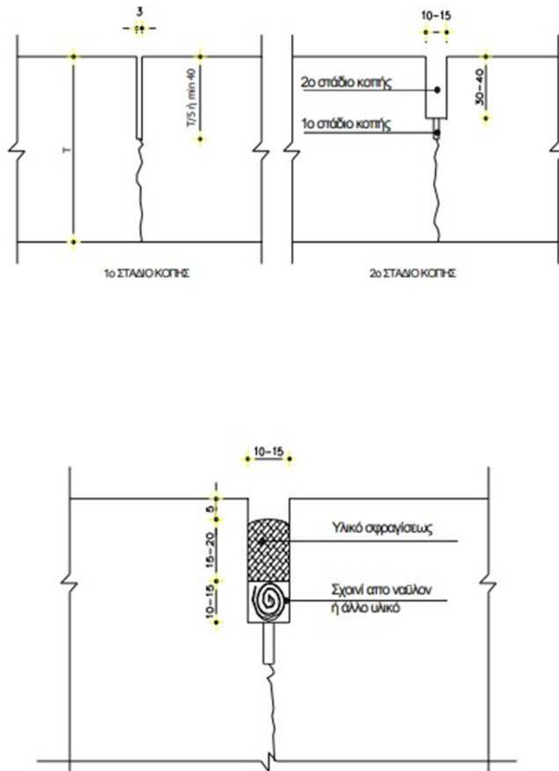
Εικόνα 1: Στάδια διαμόρφωσης αρμών
